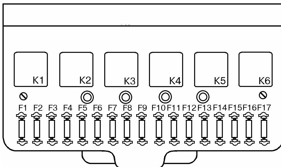
Рис.1 Расположение реле и предохранителей в монтажном блоке 2105 с пальчиковыми предохранителями
