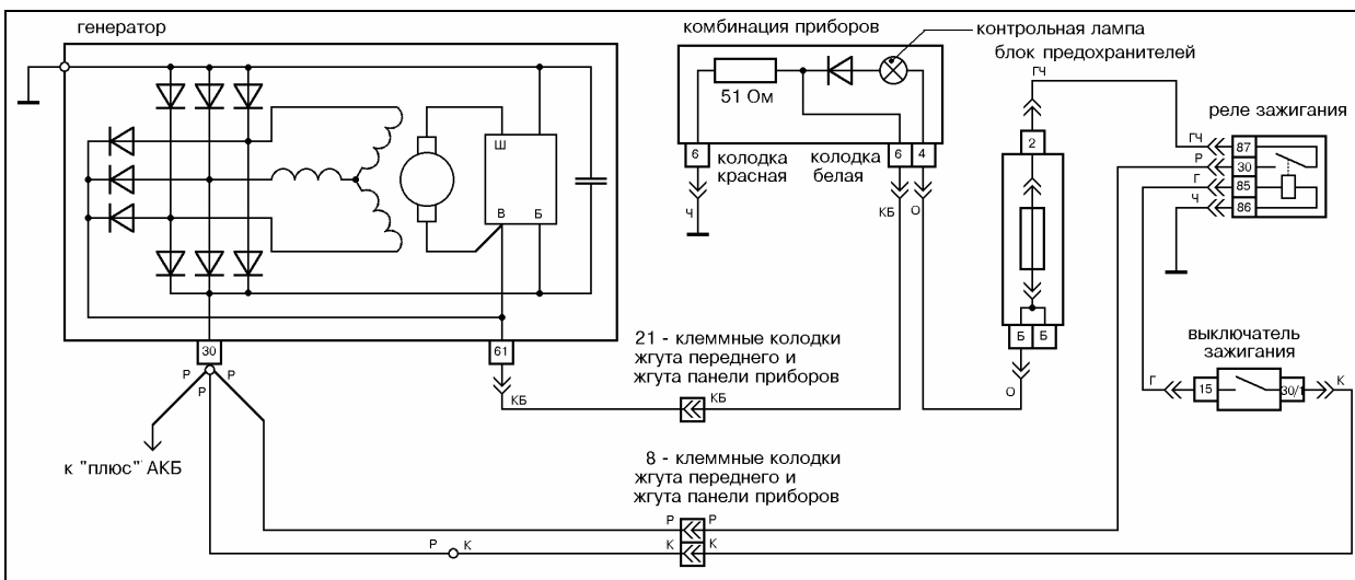
Рис.18 Схема электрических соединений генератора 21213-3701010 на а/м ВАЗ-21213.
