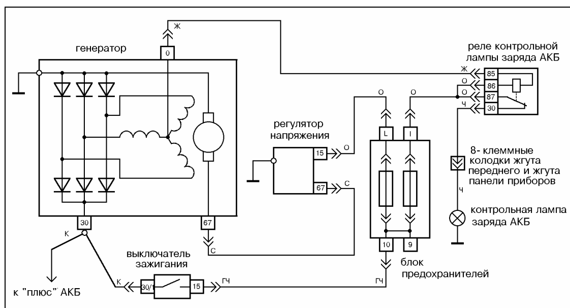
Рис.15 Схема электрических соединений генератора 2101-3701005 на а/м ВА3-2101, 2103, 2106.
