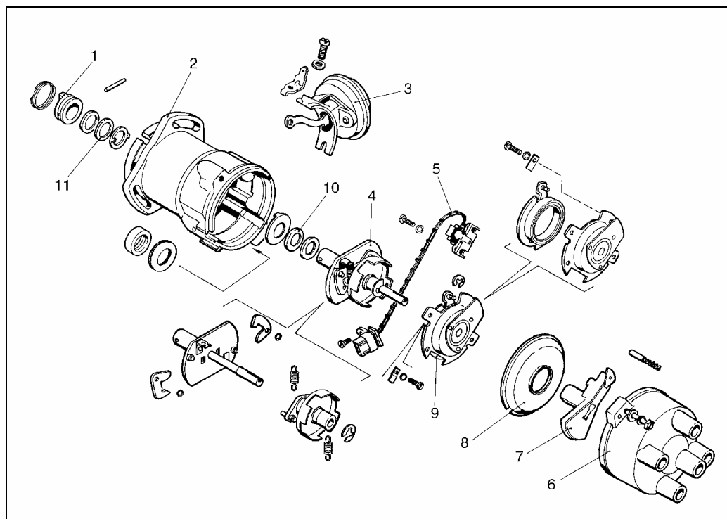
Рис.11 Детали датчика-распределителя 2108.
