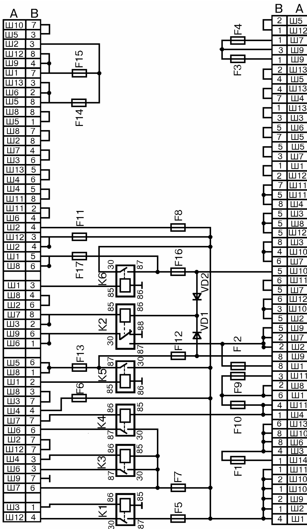
Рис. 4 Принципиальная схема внутренних соединений монтажного блока 2105.
