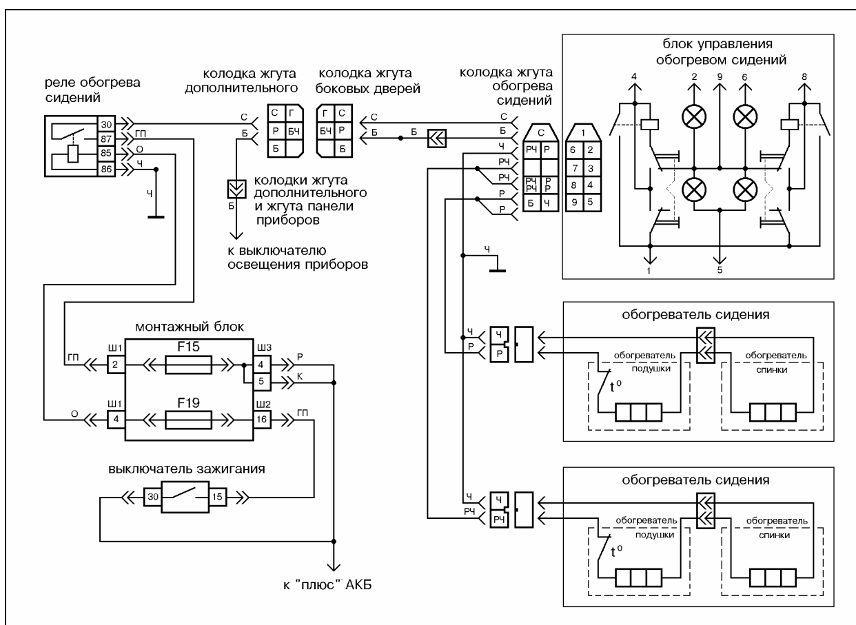
Рис.8 Схема электрических соединений обогревателя сидений на а/м VA3-2110.
