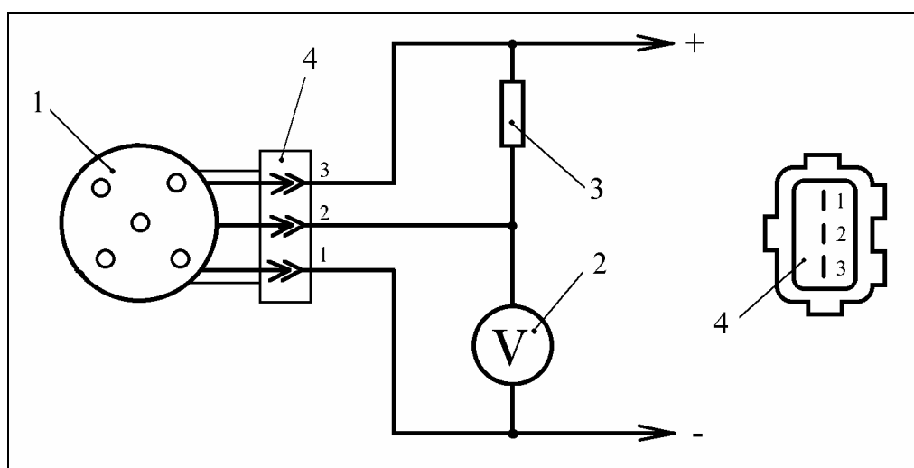
Рис.20 Схема проверки датчика.
