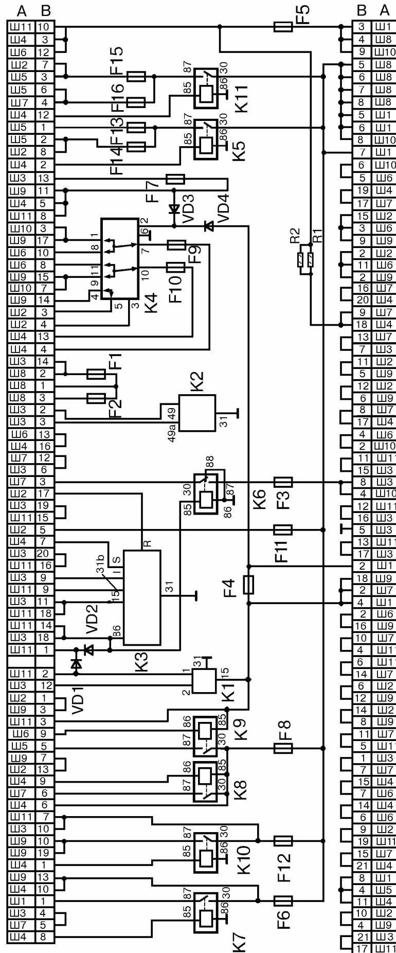
Рис. 7. Принципиальная схема внутренних соединений монтажного блока 2108.
