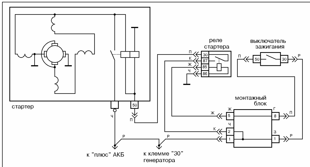
Рис.13 Схема электрических соединений стартера 2101-3708000-02 на а/м ВАЗ-2104, 2105, 2107.
