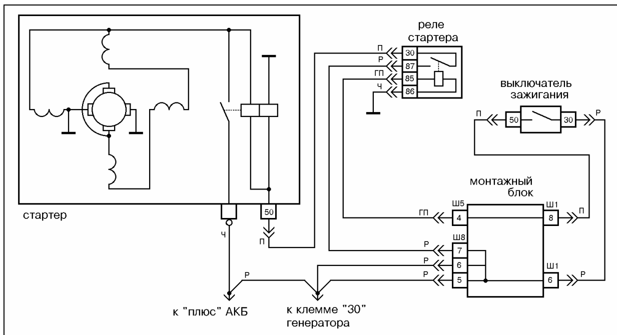
Рис.15 Схема электрических соединений стартера 2108-3708010 на а/м ВАЗ-2108, 2109, 21099.
