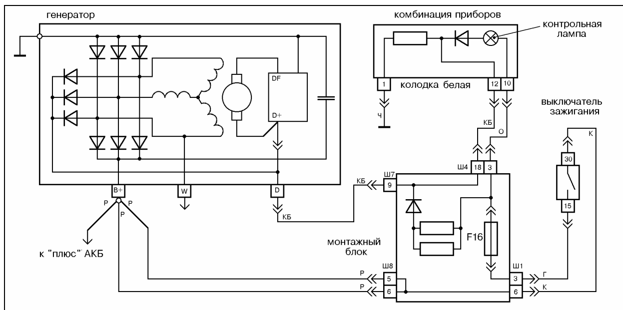
Рис.21 Схема электрических соединений генератора 2112-3701010 на а/м ВА3-2115.
