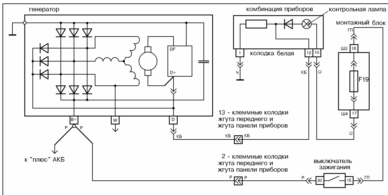
Рис.20 Схема электрических соединений генератора 2112-3701010 на а/м ВА3-2110, 2111, 2112.
