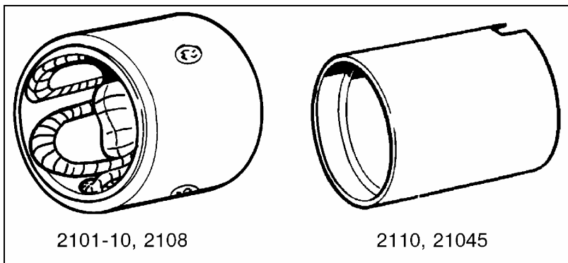
Рис.7 Корпус статора.
