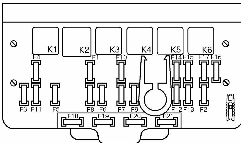
Рис.2 Расположение реле и предохранителей в монтажном блоке 2105 с ножевыми предохранителями
