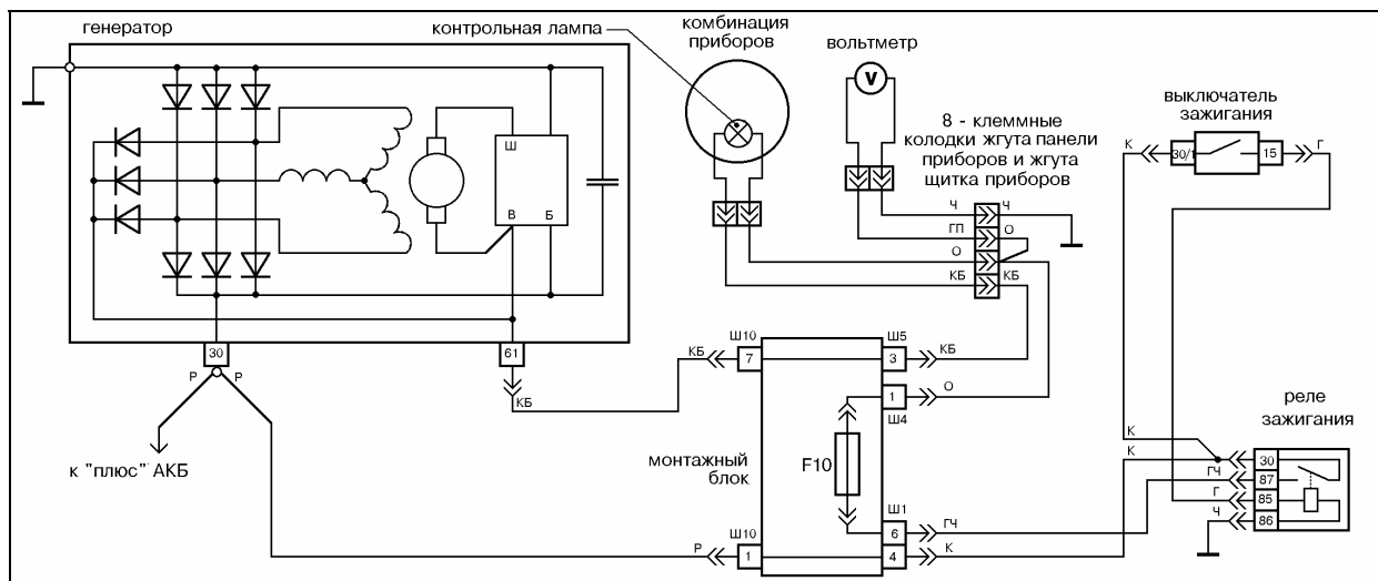
Рис.16 Схема электрических соединений генератора 2108-3701010 на а/м ВАЗ-2104, 2105.
