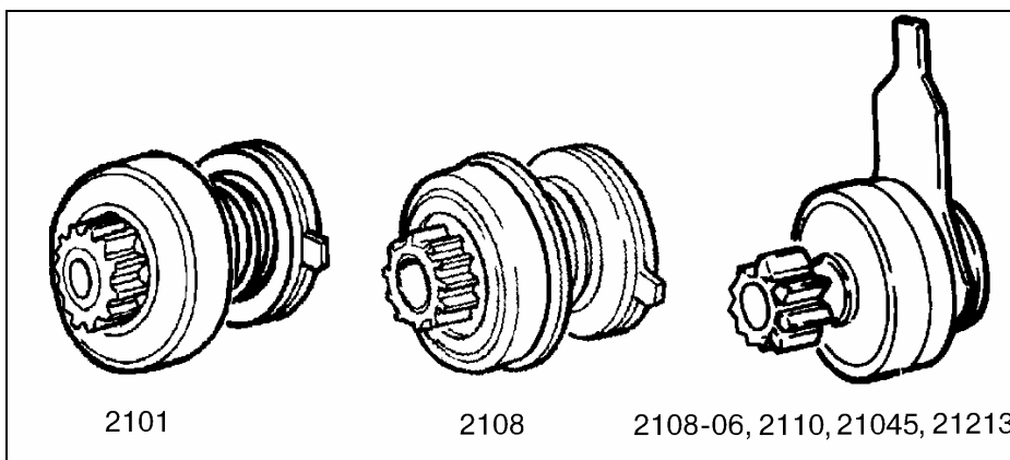
Рис.5 Привод.
