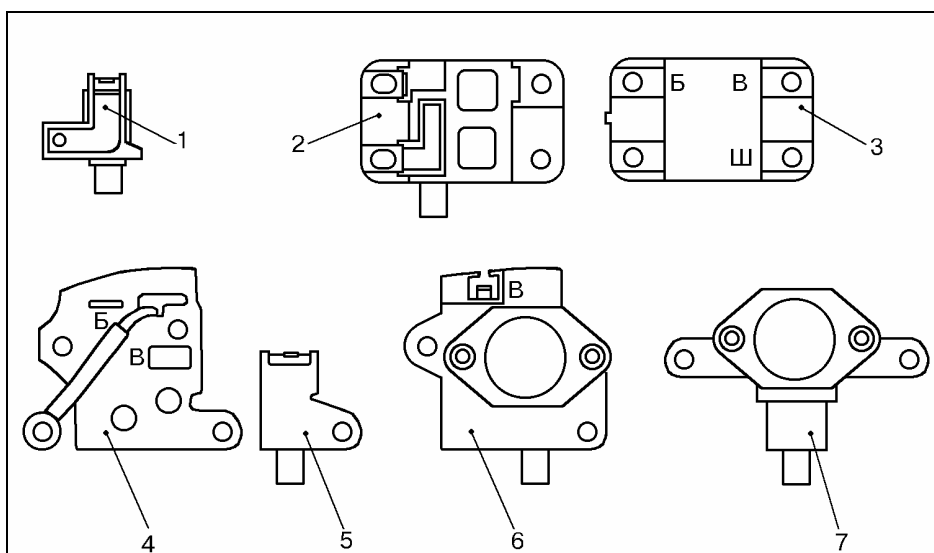
Рис.9 Регуляторы напряжения и щеткодержатели (вид спереди).
