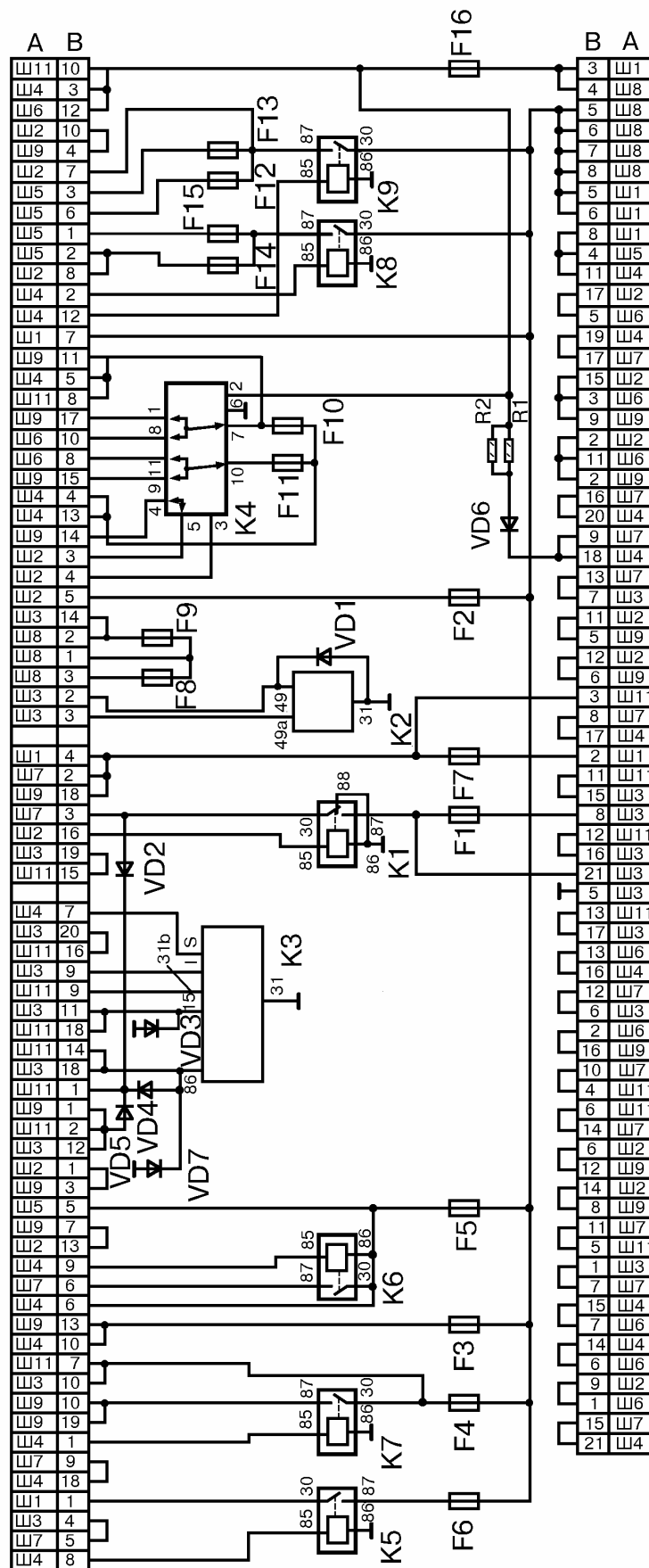
Рис. 15. Принципиальная схема внутренних соединений монтажного блока 2114.
