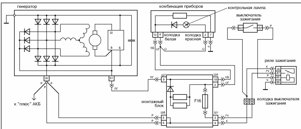
Рис.19 Схема электрических соединений генератора 2108-3701010 на а/м ВАЗ-2108, 2109, 21099 с монтажным блоком 2114-3722010.
