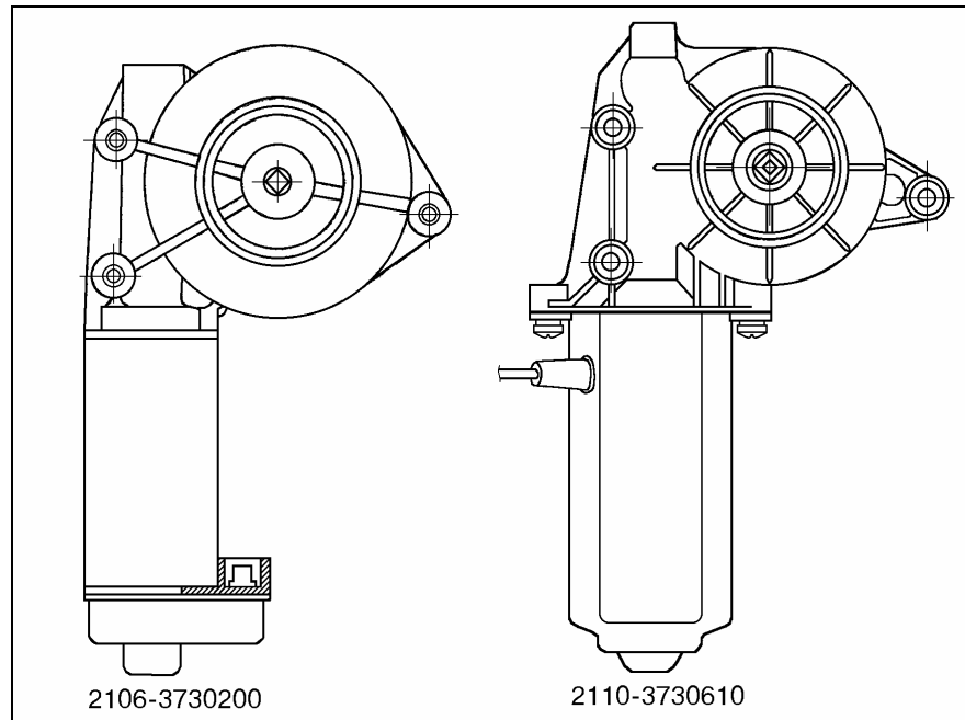
Рис.1 Моторедукторы электростеклоподъемников.
